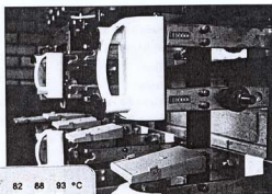
Mini rubans à 6 températures ici en utilisation sur les jeux de barres électriques.
