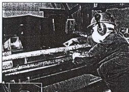
Indicateur recouvert pour vérifier la température de vulcanisation à British Steel Strip Products.
